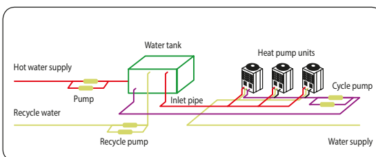
СХЕМА ГРУППОВОГО МОНТАЖА НАРУЖНЫХ БЛОКОВ RSJ НА ОБЩИЙ БАК
