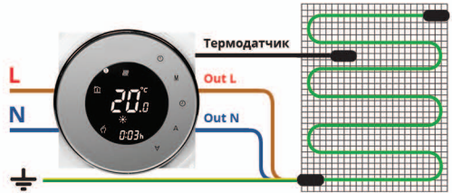
Мал. 3. Схема підключення нагрівального мата ThermoGreen™
