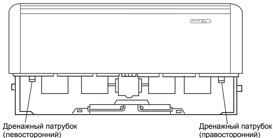
Рисунок 5. Модель AC282-482MFERA
