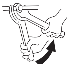
Затягивание гайки с помощью двух ключей
