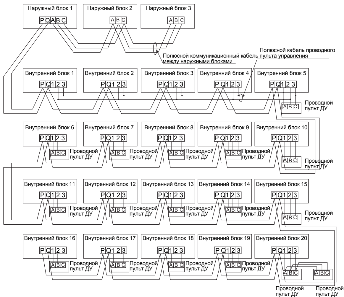
Схема подключения межблочных коммуникационных кабелей
