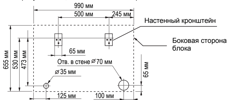
Модель AC092-242MCERA
