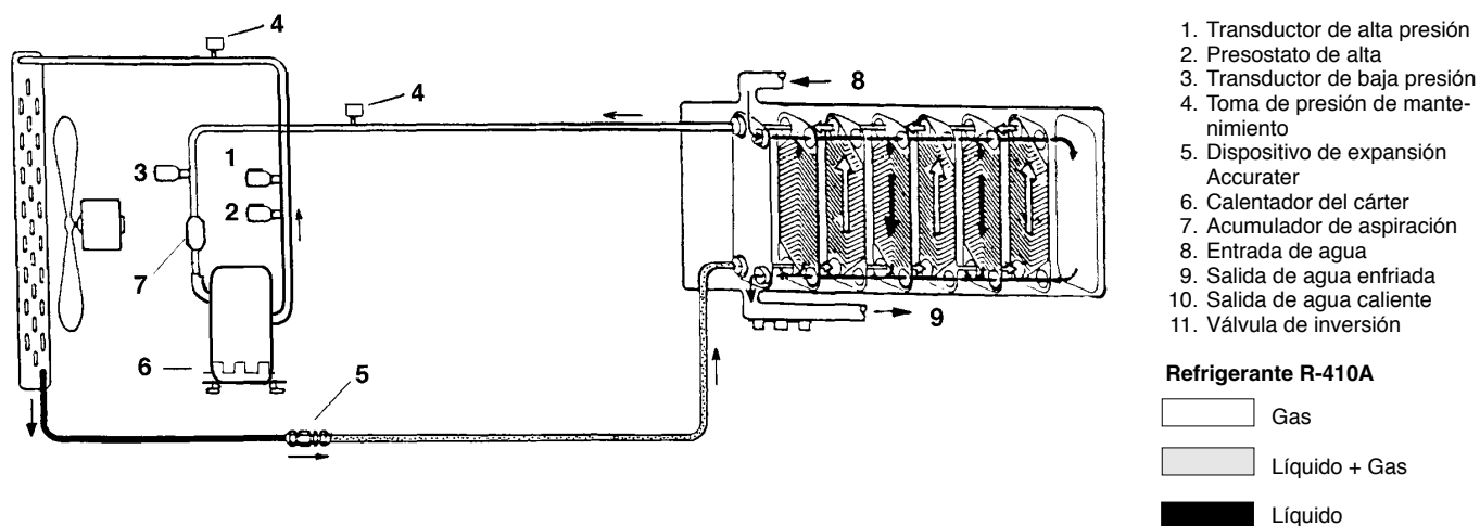
Diagrama de flujo para unidades sólo refrigeración
