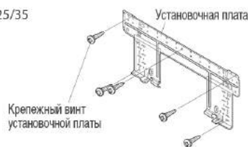
FTYN 20/25/35 (АЛЬТЕРНАТИВНЫЙ ВАРИАНТ УСТАНОВКИ ПЛАСТИНЫ)
