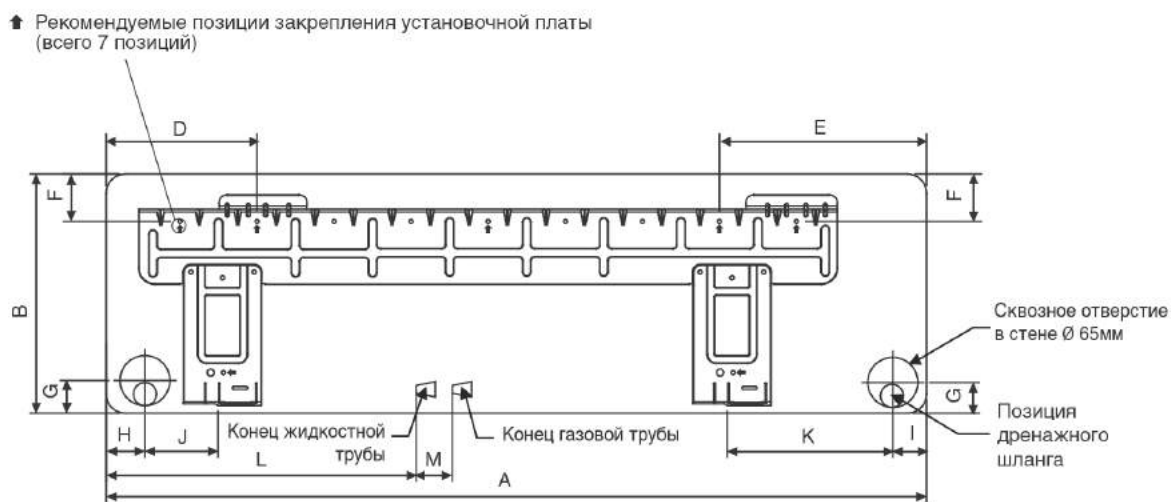
МОНТАЖНАЯ ПЛИТА 50/60
