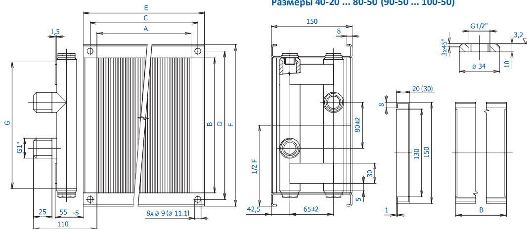
Рис. 5 Размеры водяных обогревателей SWH.
