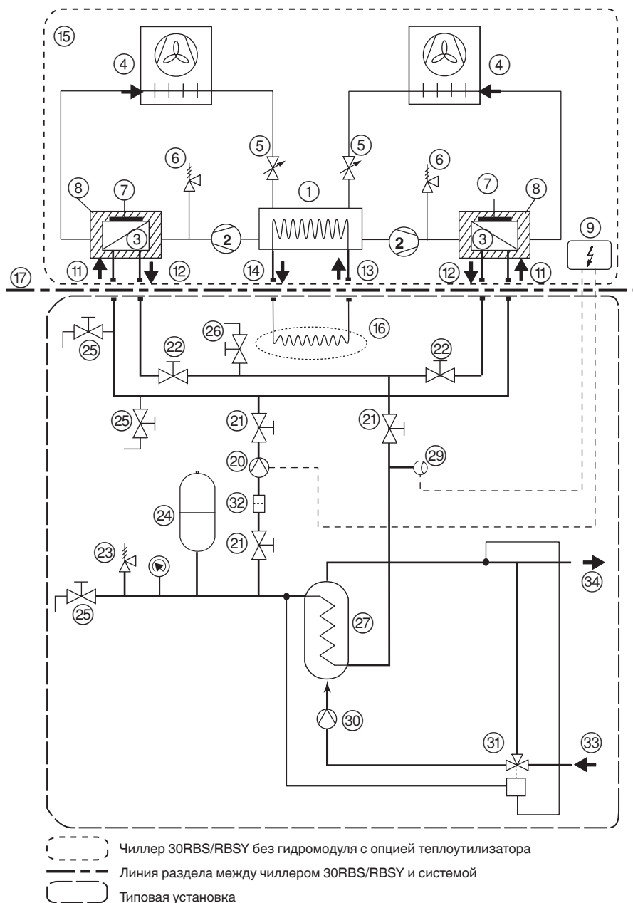
Типовая схема установки двухконтурных чиллеров с опцией теплоутилизатора
