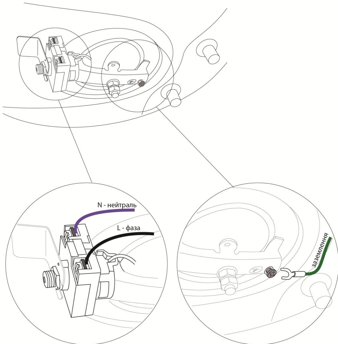
Рис. 6 – Підключення живлення.
