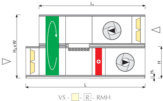
Типоразмеры VS 21÷650
