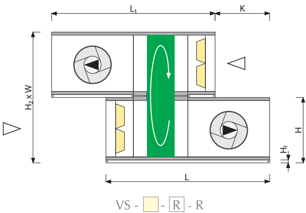
Типоразмеры VS 21÷650
