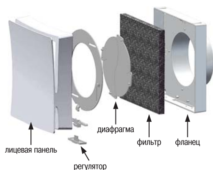
Конструкция внутренней решетки
